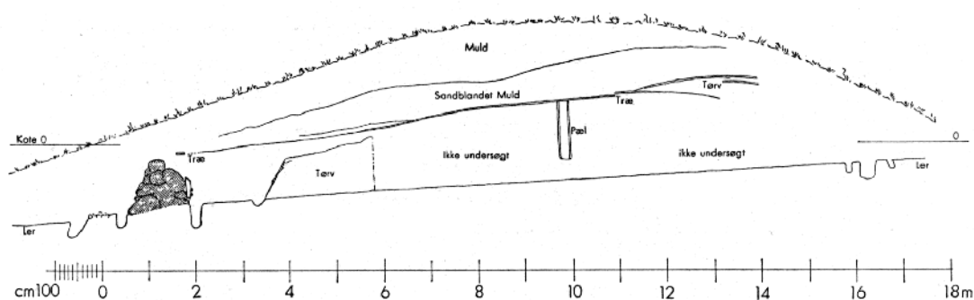
Figur 2. Snit gennem ringvolden i afsnittet mod nordvest (Nørlund 1948).
